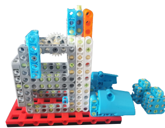
图 2-3 能量块被取下
